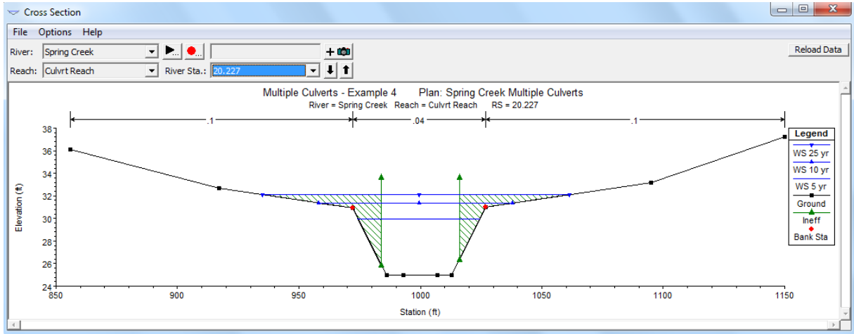
Şekil 10 20.238 ve 20.227 kesitleri
