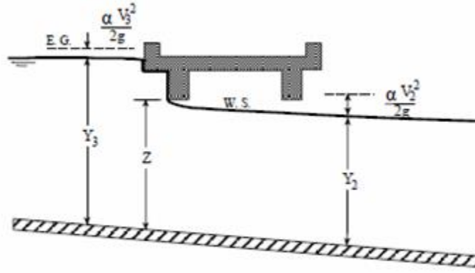
Şekil 2.4 Kapak akımı şeklinde basıncılı köprü
