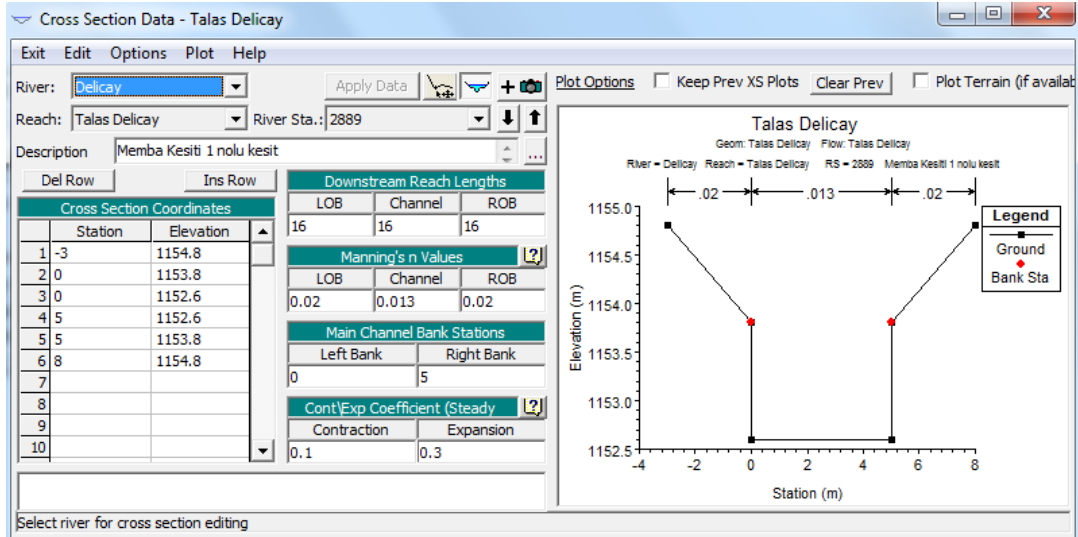
(a) Delicay deresi memba kesiti
