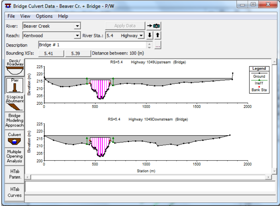
Şekil 10 Köprü görünüşü
