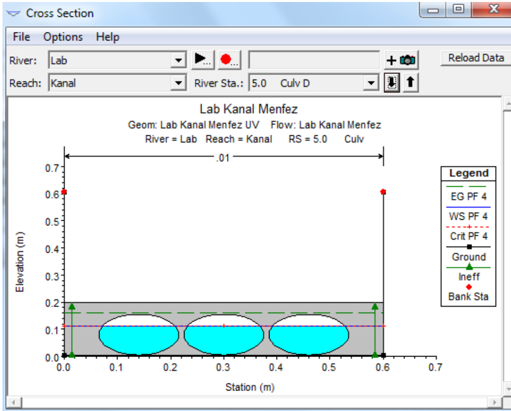
Şekil 25 (b) PF4 menfez mansap kesiti
