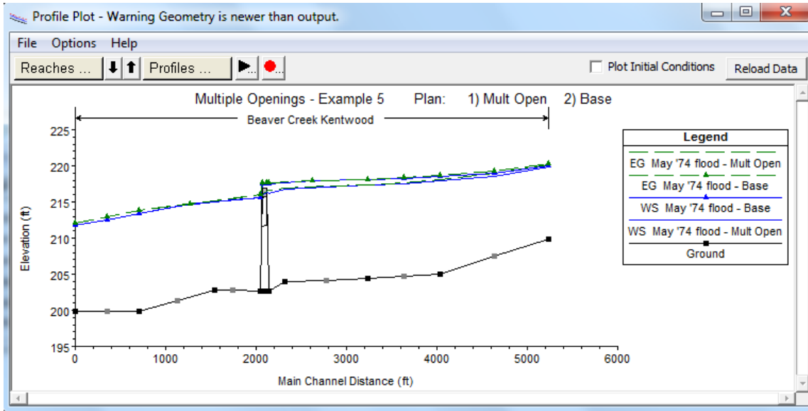
Şekil 12 Üçüncü profile ait tek ve çoklu açıklık su yüzü profillerinin karşılaştırılması
