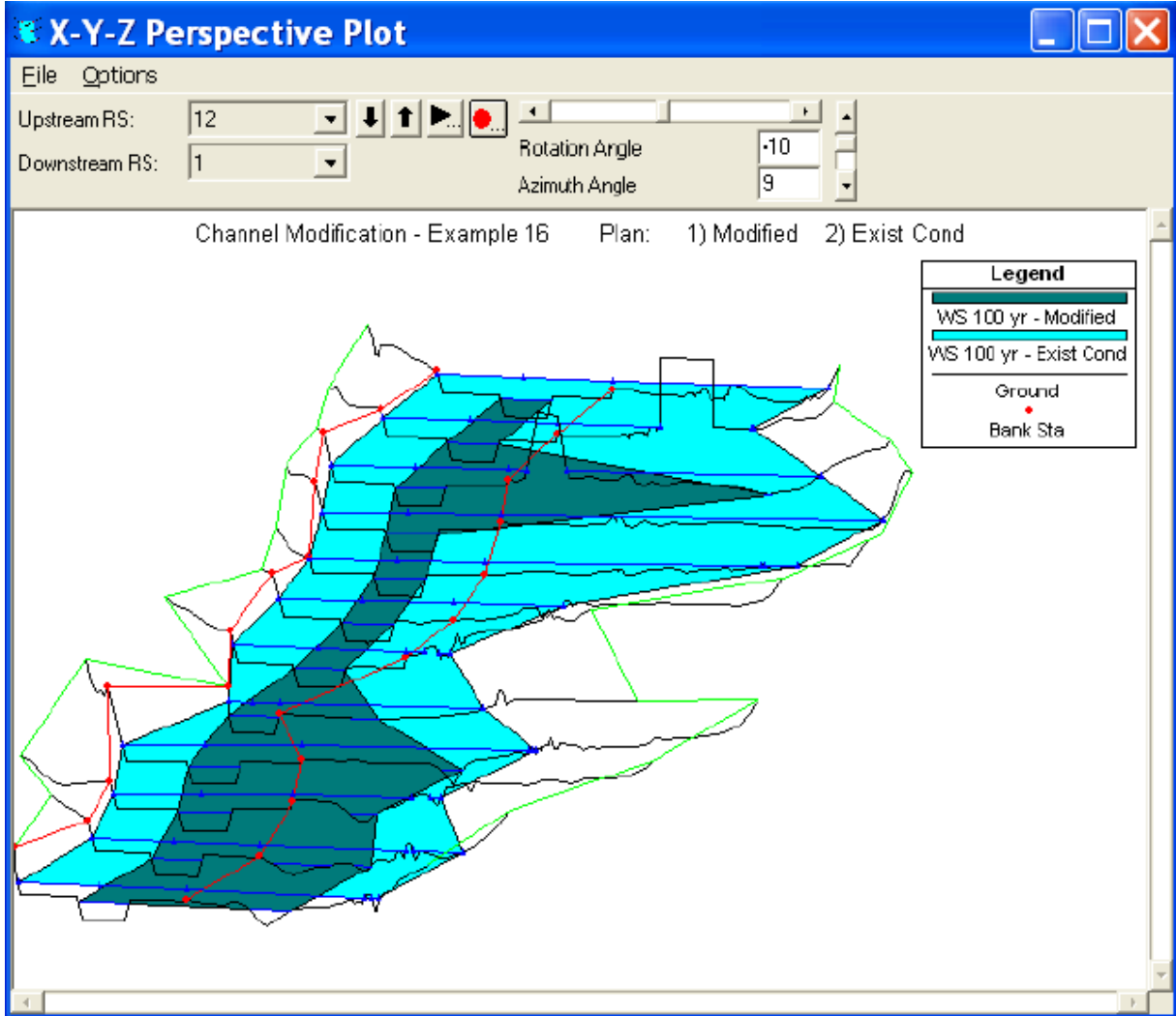
Şekil 9 Üç boyutlu görünüm
