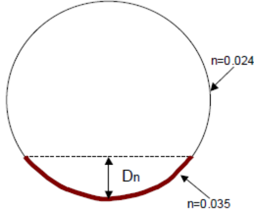
Şekil 3.10 Farklı pürüzlülüğe sahip menfez kesiti
