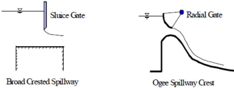
Şekil 5.1 Kesit üzerinde kapaklı dolu savak ve kapaksız savak örneği
