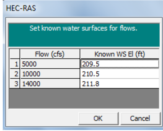
Şekil 16 Sınır şartları için bilinen su yüzü kotları
