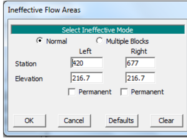
Şekil 11 Etkisiz akım bölgeleri, 5.41 nolu kesit için
