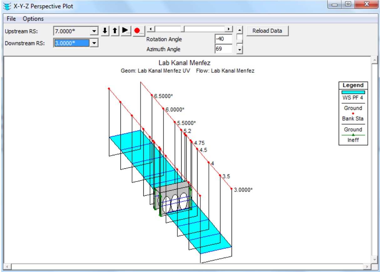
Şekil 27 PF4 için kanal 3.0-7.0m arası üç boyutlu görünüm
