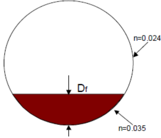
Şekil 3.11 Kısmi engel dolu menfez
