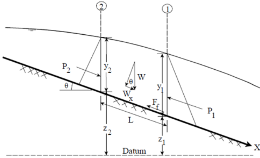
Şekil 1.5 Momentum yöntemindeki büyüklükler
