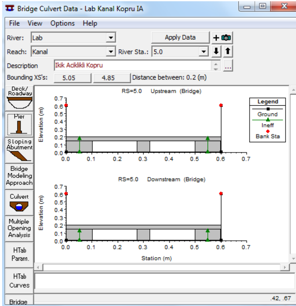
Şekil 37 İki açıklıklı köprü memba ve mansap kesit görünüşleri
