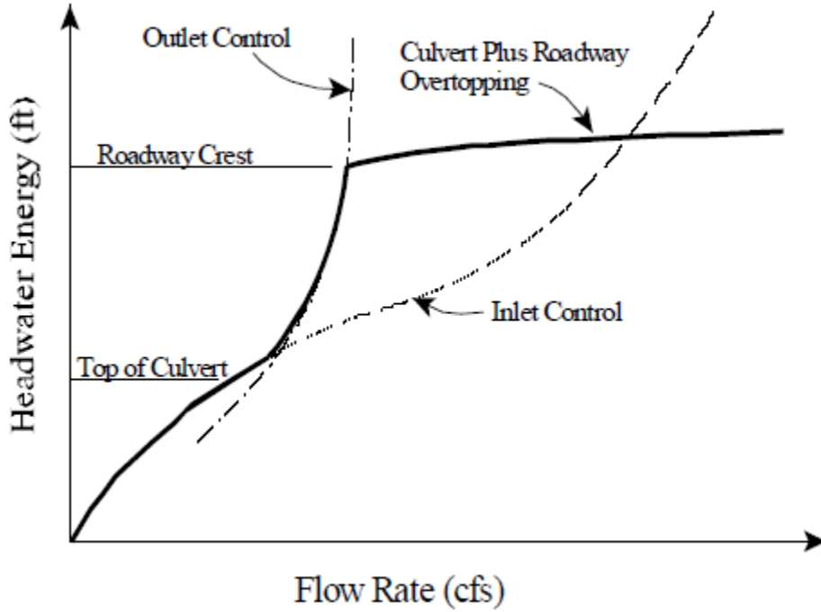
Şekil 3.8 Menfez performans eğrisi, yol seviyesinin aşılması hali
