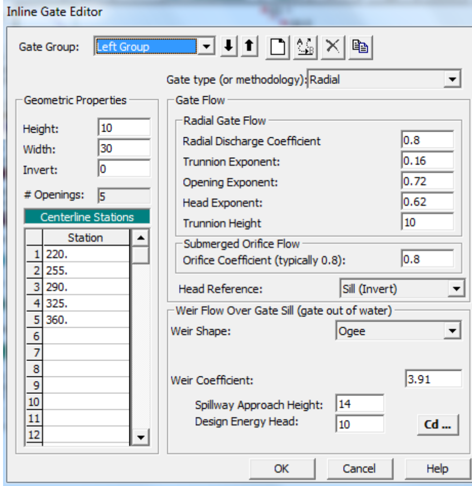
Şekil 6 Kapak penceresi
