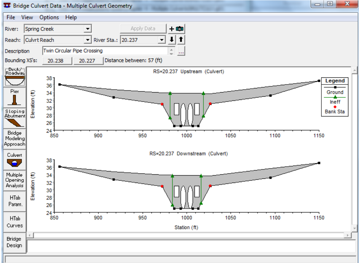
Şekil 4 Kutu ve Dairesel Menfezler, 20.237 kesitinde
