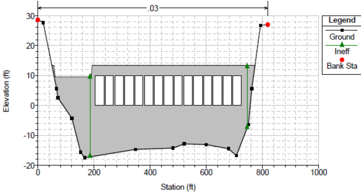
Şekil 5.1 Kesit üzerinde kapaklı dolu savak ve kapaksız savak örneği
