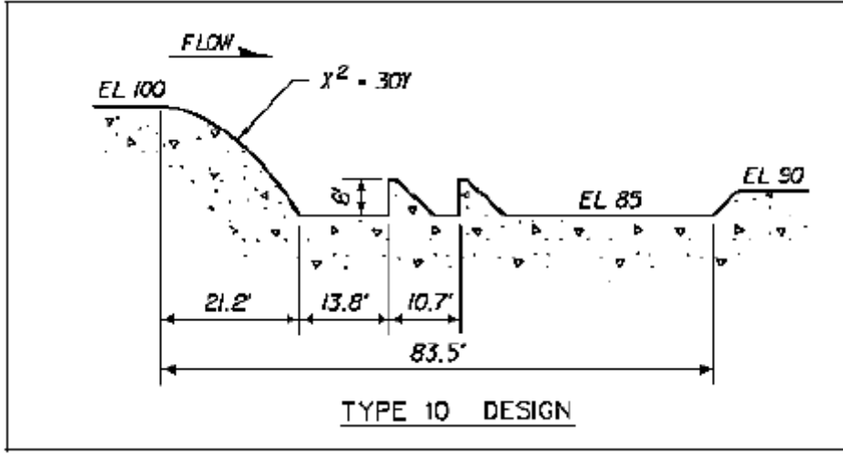
Şekil 5.14 WES raporu kesit 13
