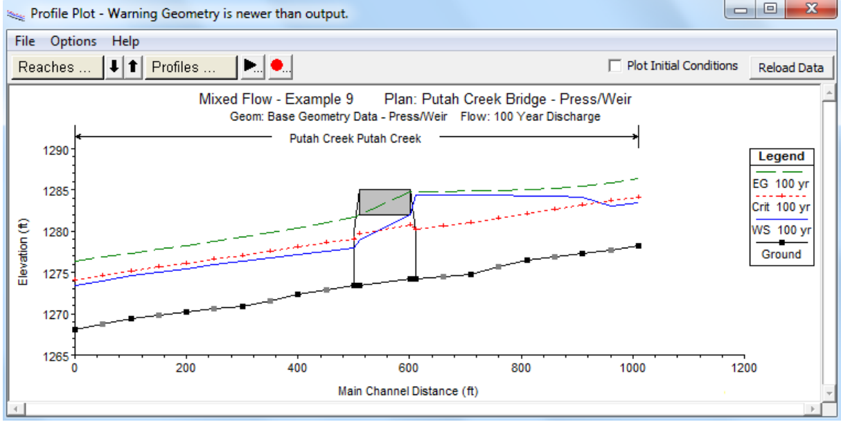
Şekil 18 Basınçlı savak akımı analizinde su yüzü profilleri
